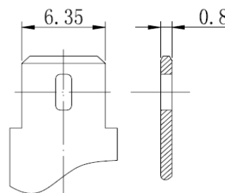
Клеммы
