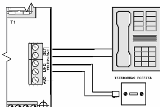
Рис. 14 Подключение телефонной линии и дополнительных устройств
