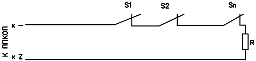
Рис.6 Формирование шлейфов с одним оконечным резистором из нормально замкнутых датчиков
