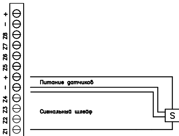
Рис. 2 Подключение датчиков к ППКОП «Captain-i»
