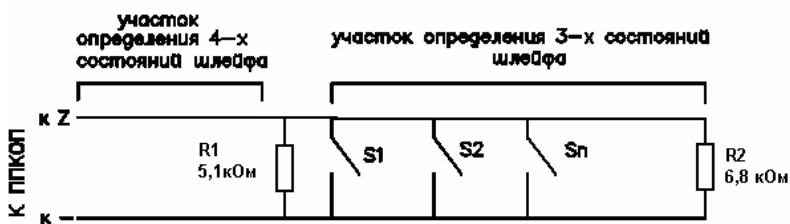
Рис. 35 Участки определения состояний зон
