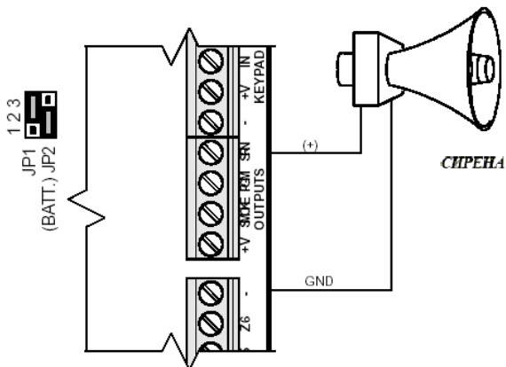
Рис. 12 Подключение сирены с встроенным генератором с высоким потреблением тока
