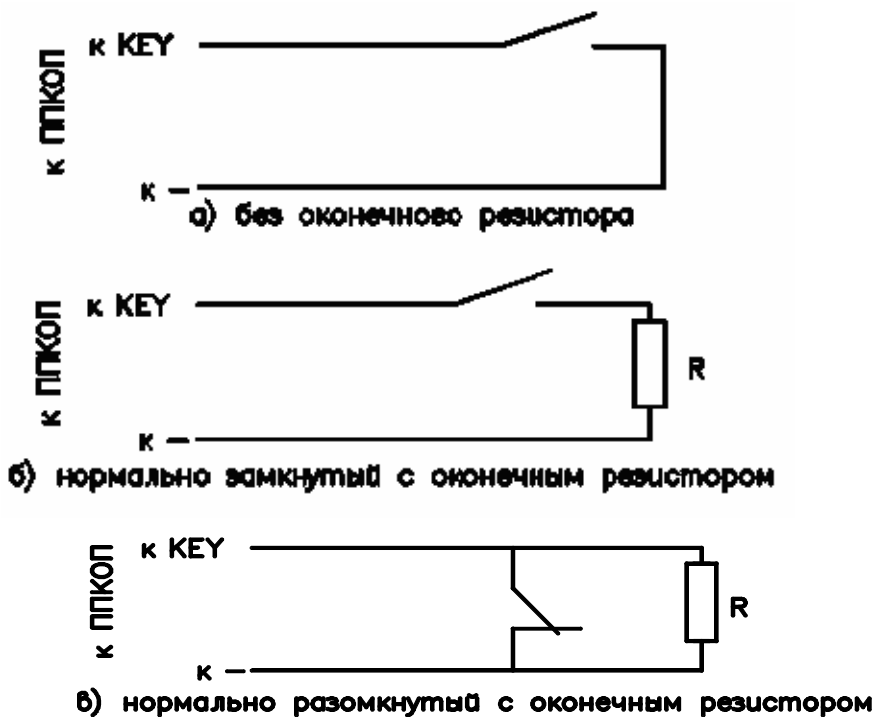
Рис. 9 Способы подключения ключа
