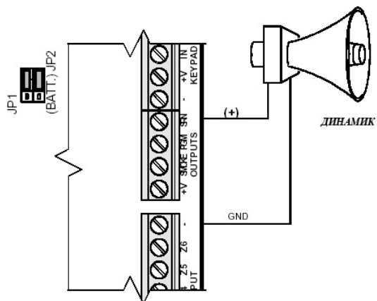
Рис. 10 Подключение сирены типа «горн»
