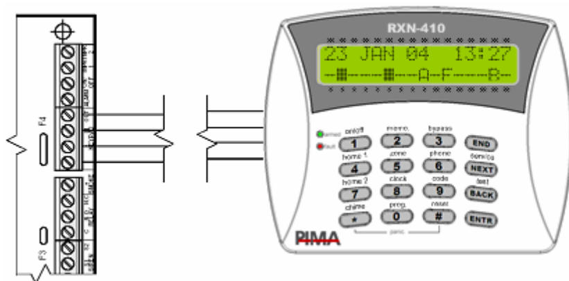
Рис. 13 Подключение клавиатур
