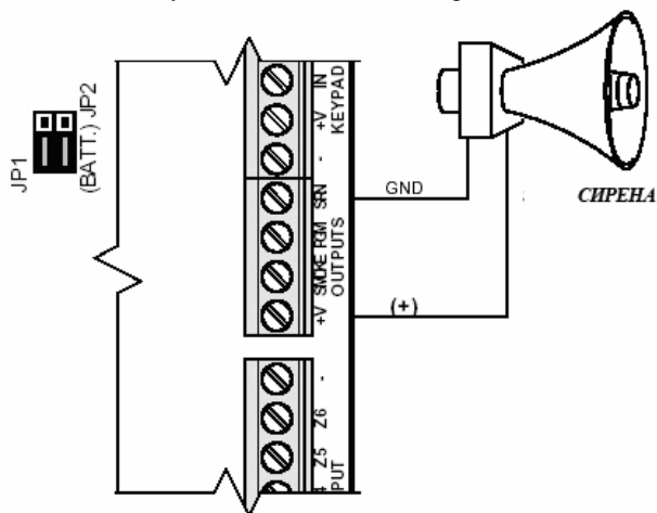
Рис. 11 Подключение сирены с встроенным генератором
