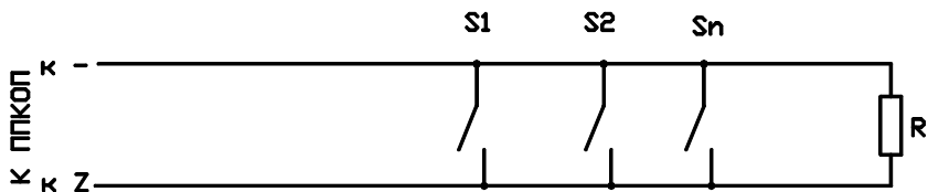
Рис.5 Формирование шлейфов с одним оконечным резистором из нормально разомкнутых датчиков
