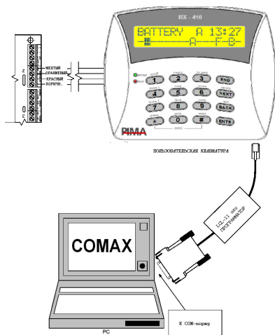
Рис. 18 Подключение для локального программирования.
