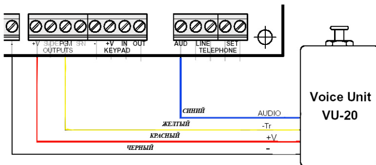
Рис. 16 Подключение голосового блока.
