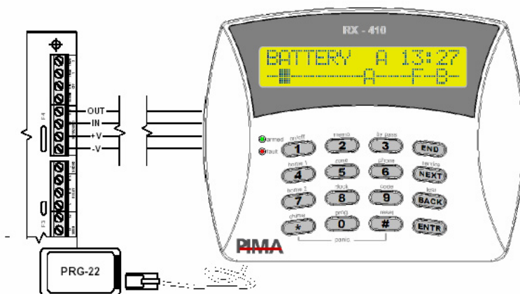
Рис. 17 Подключение программатора Для ввода программы см п. 4.16
