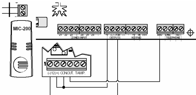
Рис.15 Подключение микрофона
