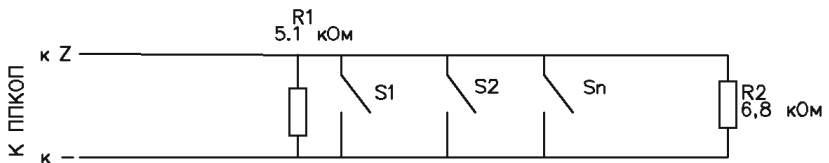
Рис. 8 Формирование шлейфа с двумя оконечными резисторами из нормально разомкнутых датчиков
