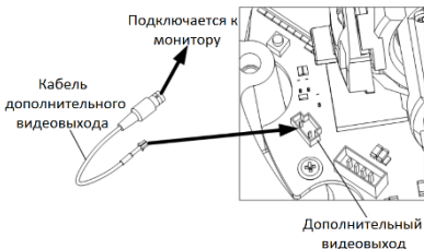
Рисунок 2-12 Подключение камеры к монитору
