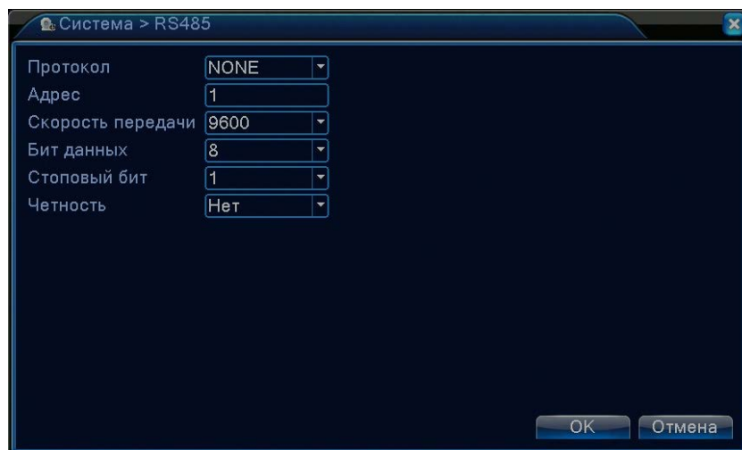
Рисунок 4.33 Конфигурация RS485 устройств в цифровом режиме.
