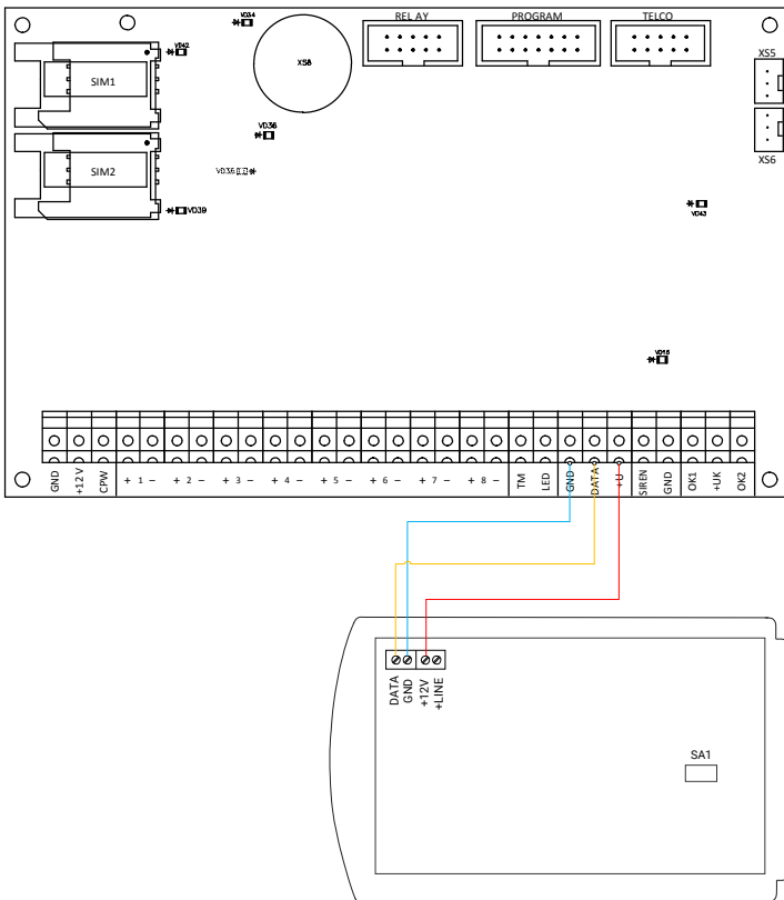
Рисунок 19. Схема подключения проводной клавиатуры
