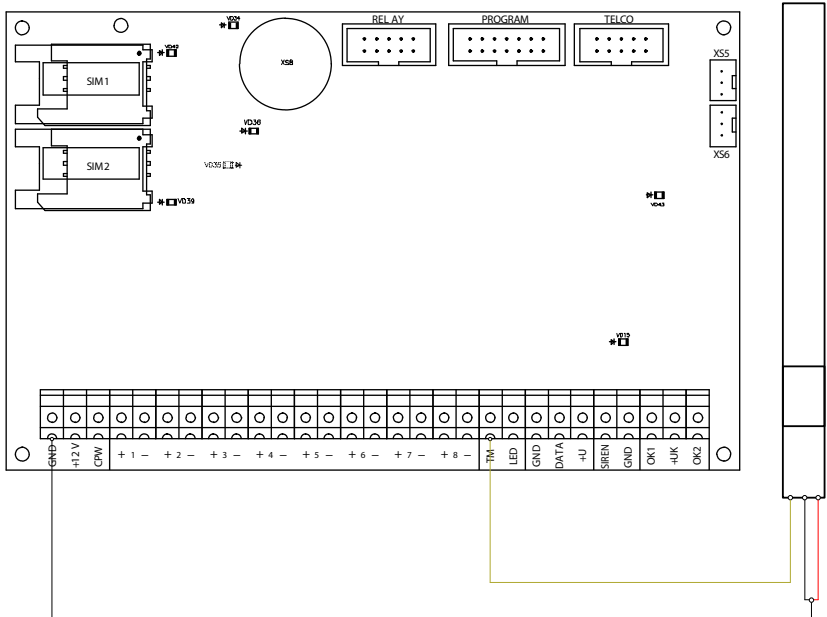
Рисунок 17. Схема подключения датчика температуры
