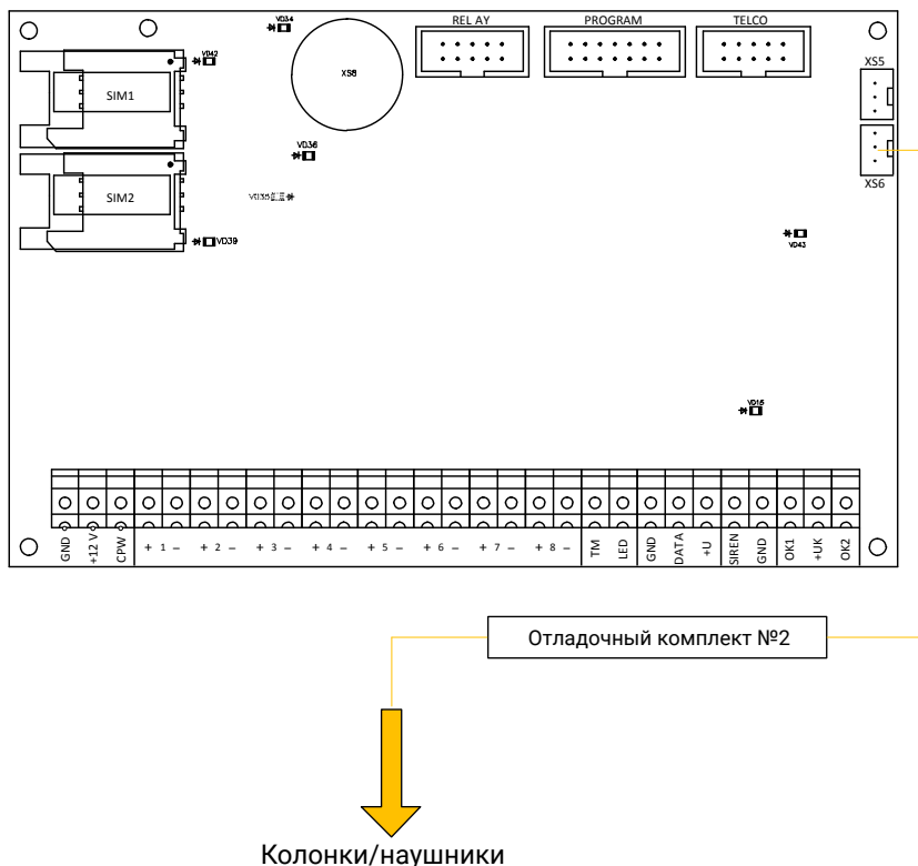
Рисунок 28. Схема подключения «Отладочного комплекта №2»
