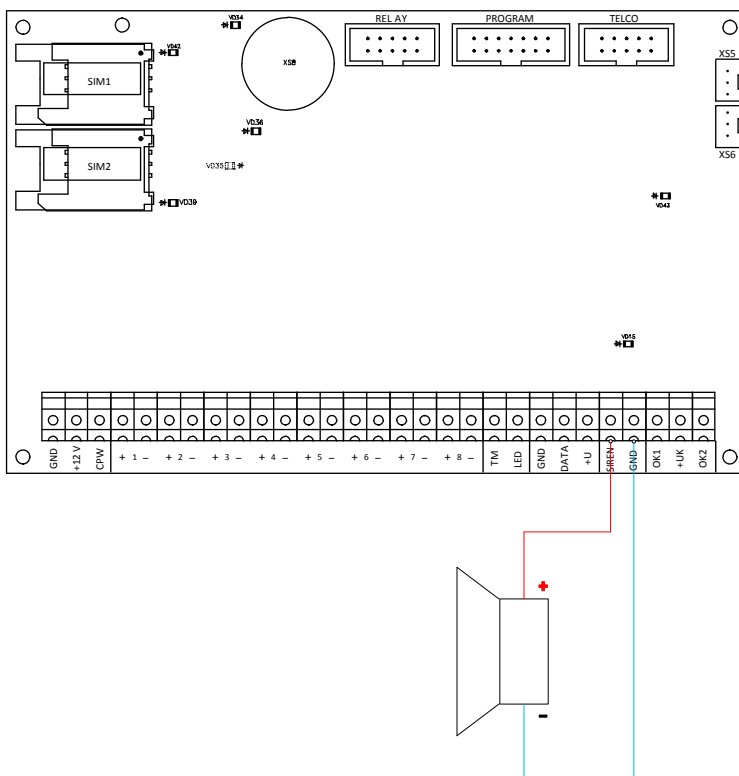
Рисунок 22. Схема подключения сирены
