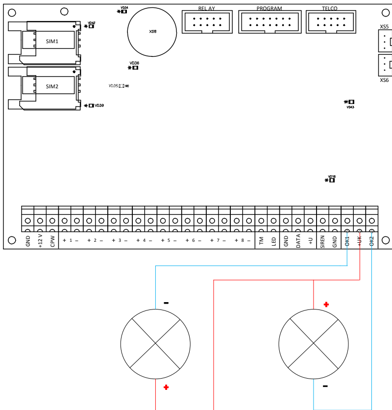
Рисунок 23. Схема подключения исполнительных устройств
