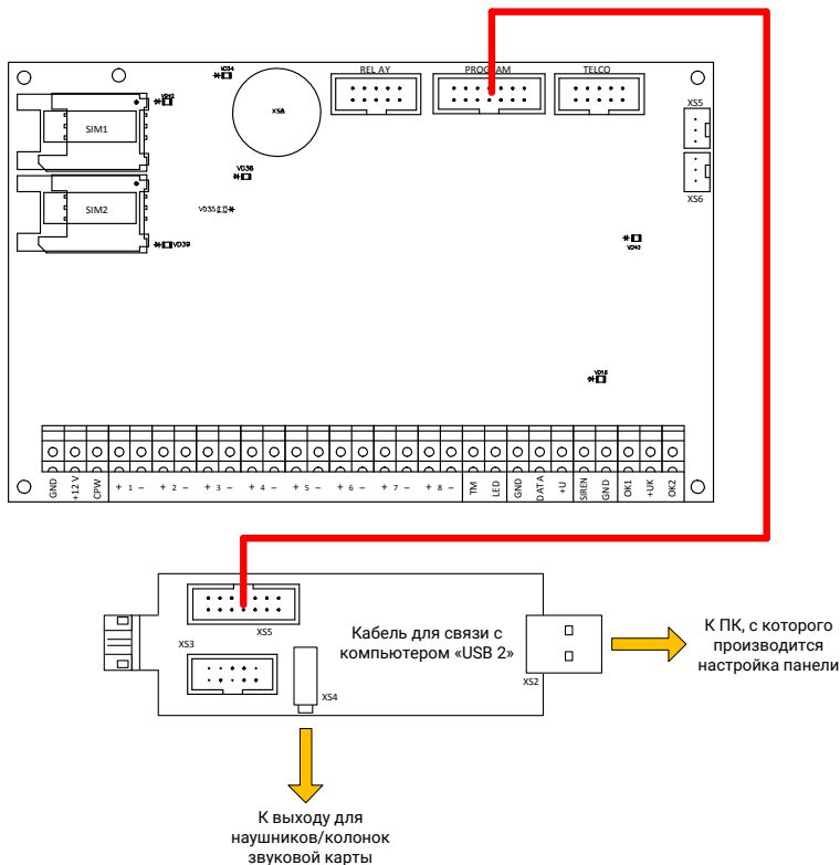
Рисунок 29. Схема подключения оборудования для записи звуков
