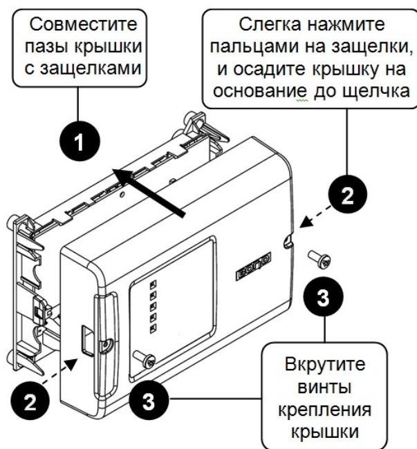
Рисунок 8. Монтаж крышки
