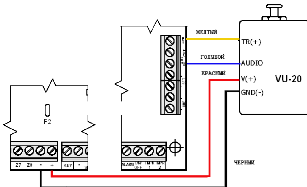
Рисунок 27 - Подключение голосового блока
