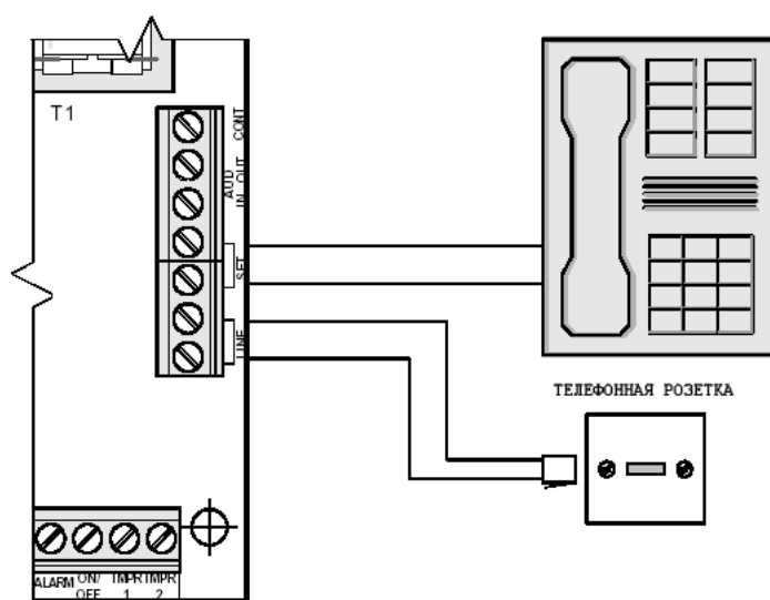
Рисунок 25 - Подключение телефонной линии и дополнительных устройств
