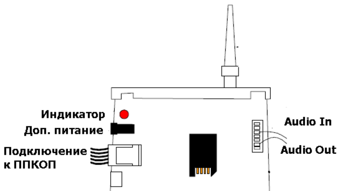
Рисунок 30 - GSM-модуль
