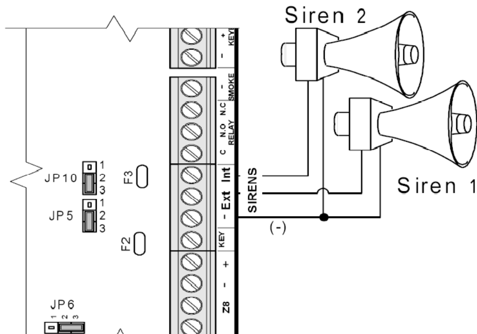
Рисунок 12 - Подключение сирены типа «горн»
