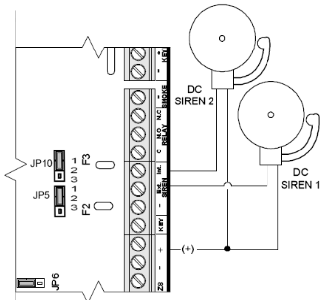
Рисунок 14 - Подключение сирены с встроенным генератором с высоким потреблением тока
