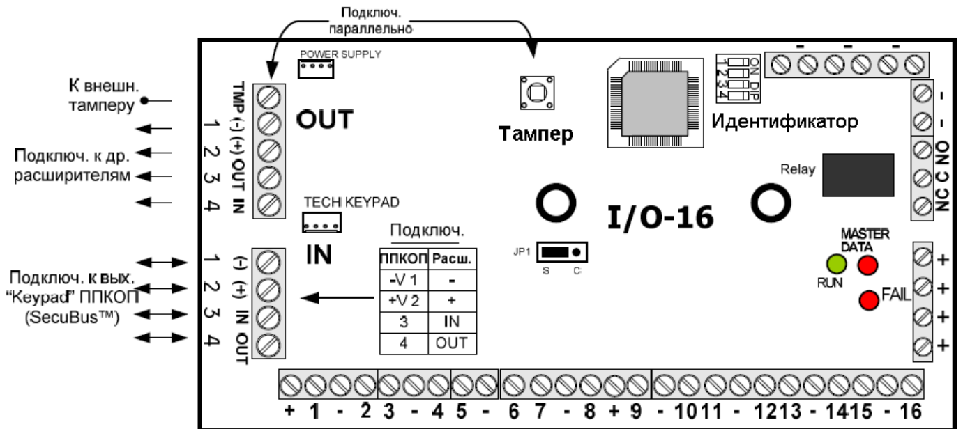
Рисунок 19 - Выносной расширитель I/O – 16
