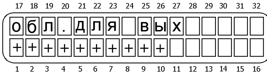
Рисунок 62 - Сопоставление областей
