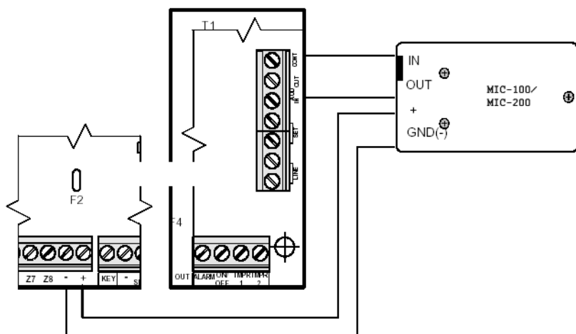
Рисунок 26 - Подключение микрофона
