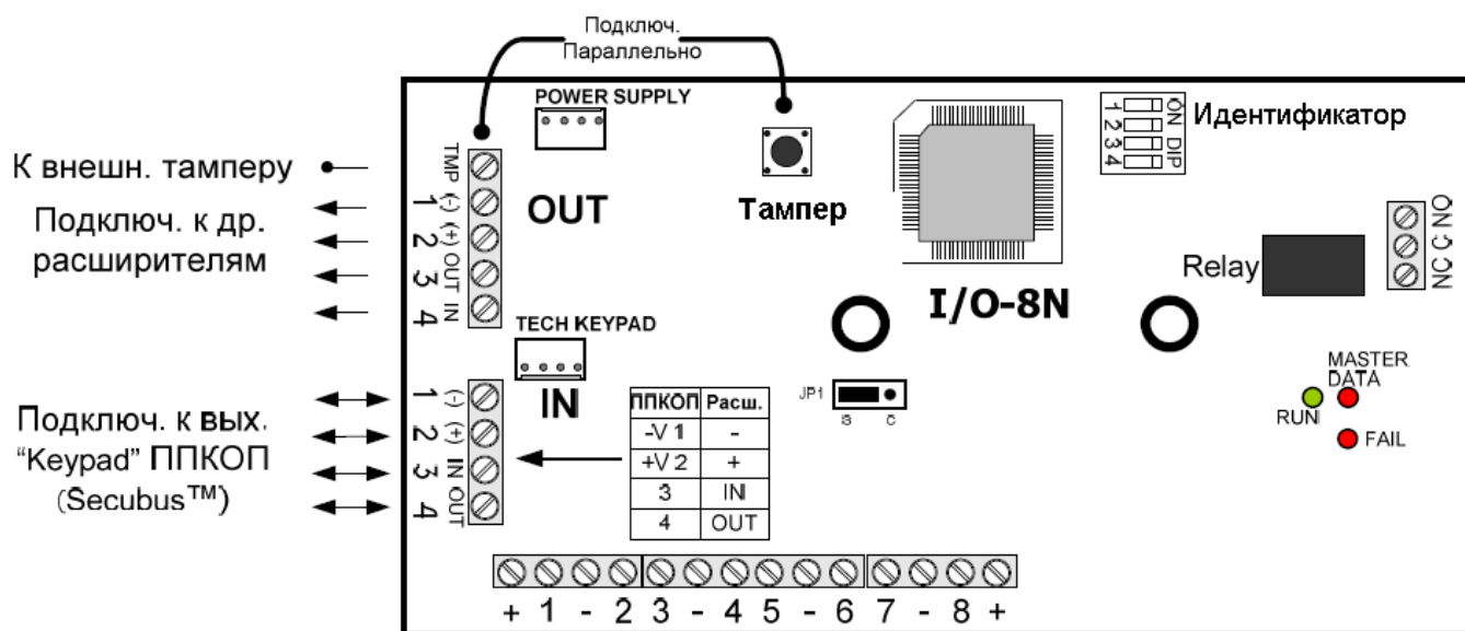
Рисунок 18 - Выносной расширитель I/O – 8N
