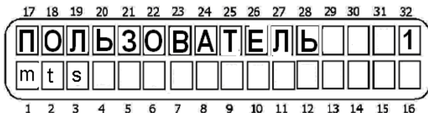
Рисунок 57 - Имя пользователя
