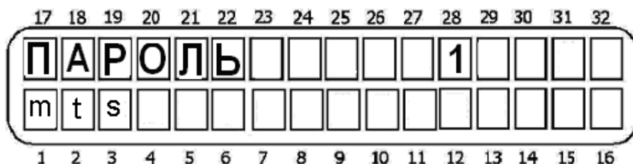
Рисунок 58 - Пароль пользователя
