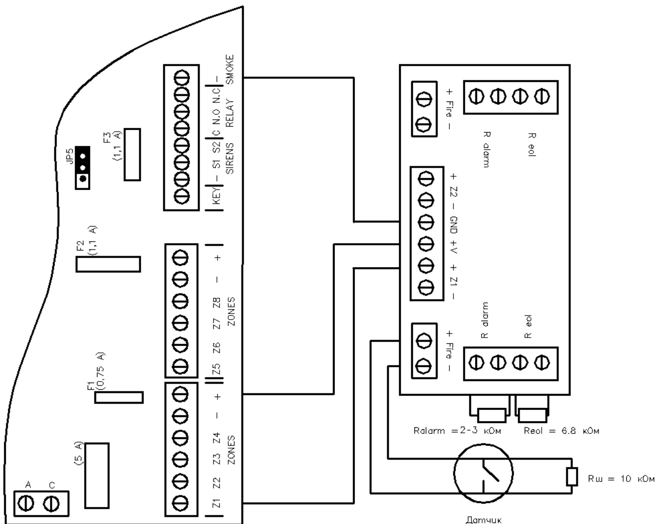
Рисунок 10 - Формирование шлейфов нормально разомкнутых пожарных датчиков при помощи ПСШ-2 со схемой подключения «два резистора в шлейфе»
