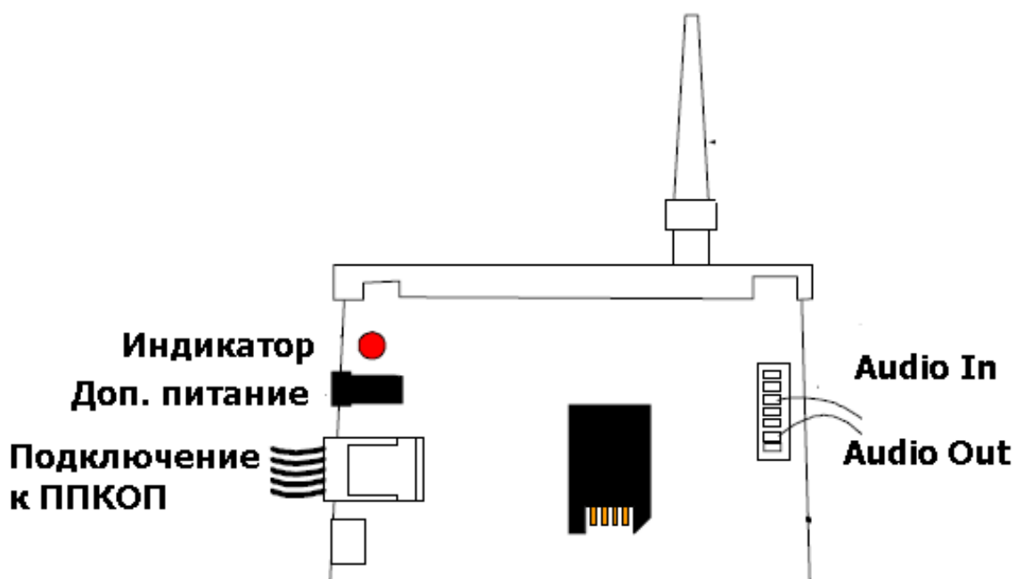
Рисунок 30 - GSM-модуль
