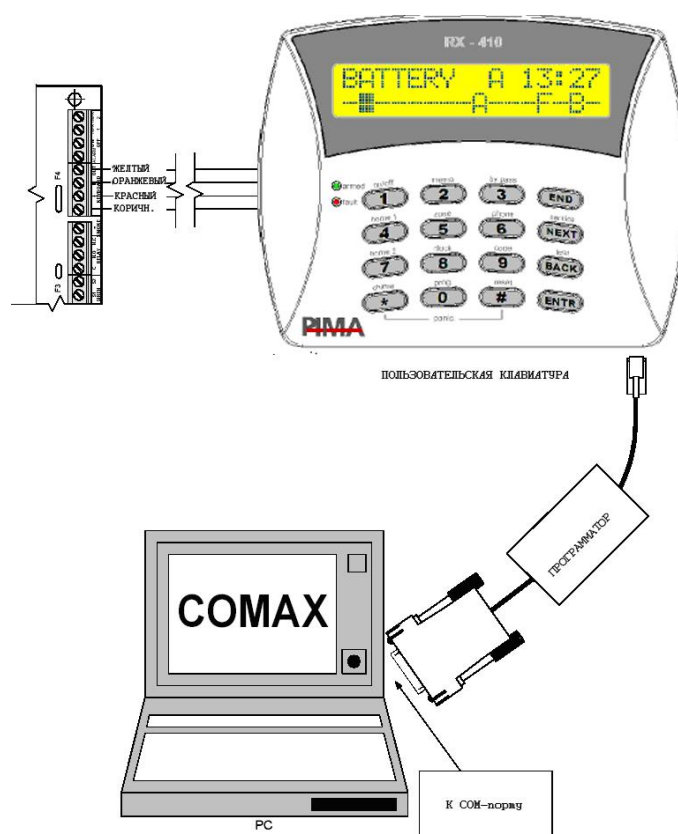
Рисунок 32 - Подключение для локального программирования.
