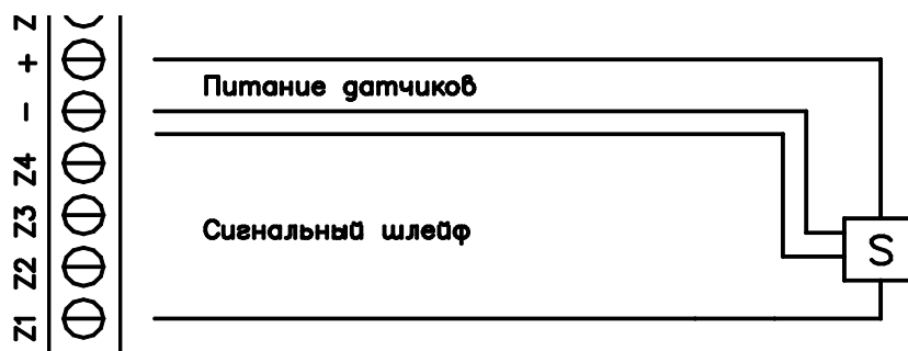
Рисунок 2 - Подключение датчиков к ППКОП «Hunter-Pro (32, 96, 144)»
